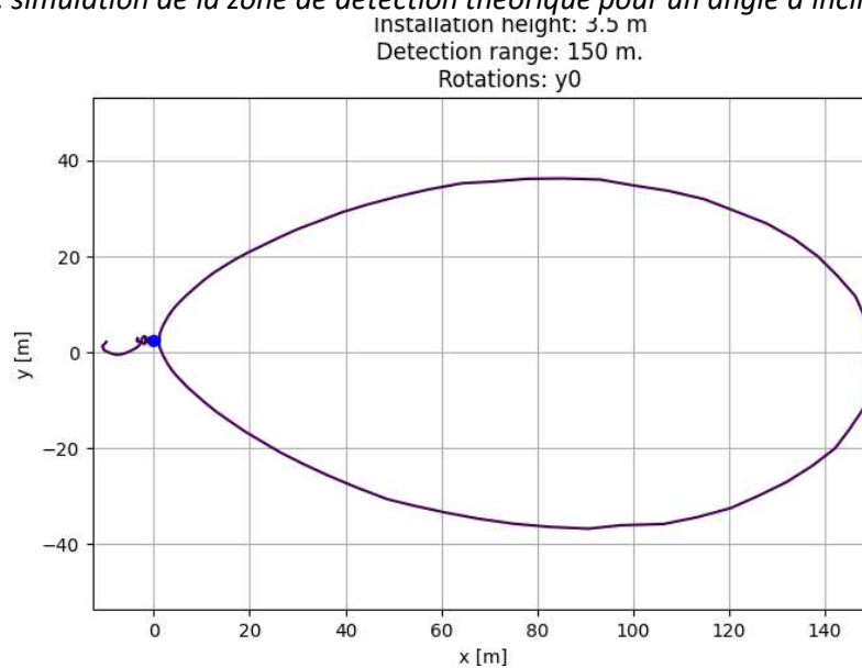
Figure 9 : simulation de la zone de détection théorique pour un angle d'inclinaison de 0^\circ
