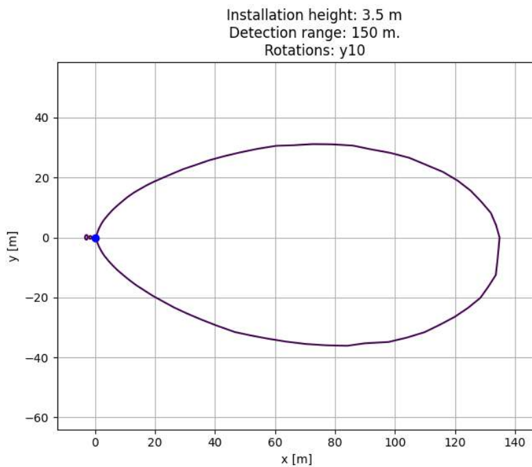
Figure 8 : simulation de la zone de détection théorique pour un angle d'inclinaison de 10^\circ
